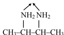
Butylenediamine(bn)
