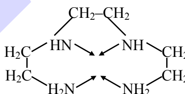
Triethylenetetraamine(trien)
