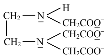
(EDTA) -3
