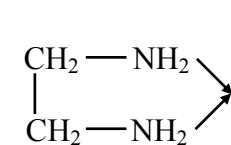
Ethylenediamine (en)
