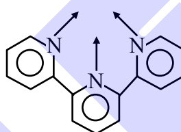
2, 2', 2''-Terpyridine (Terpy)
